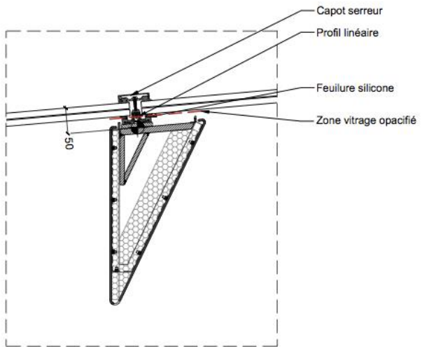
03 DETAIL SUPPORT DU VERRE ECHELLE: 1/10
