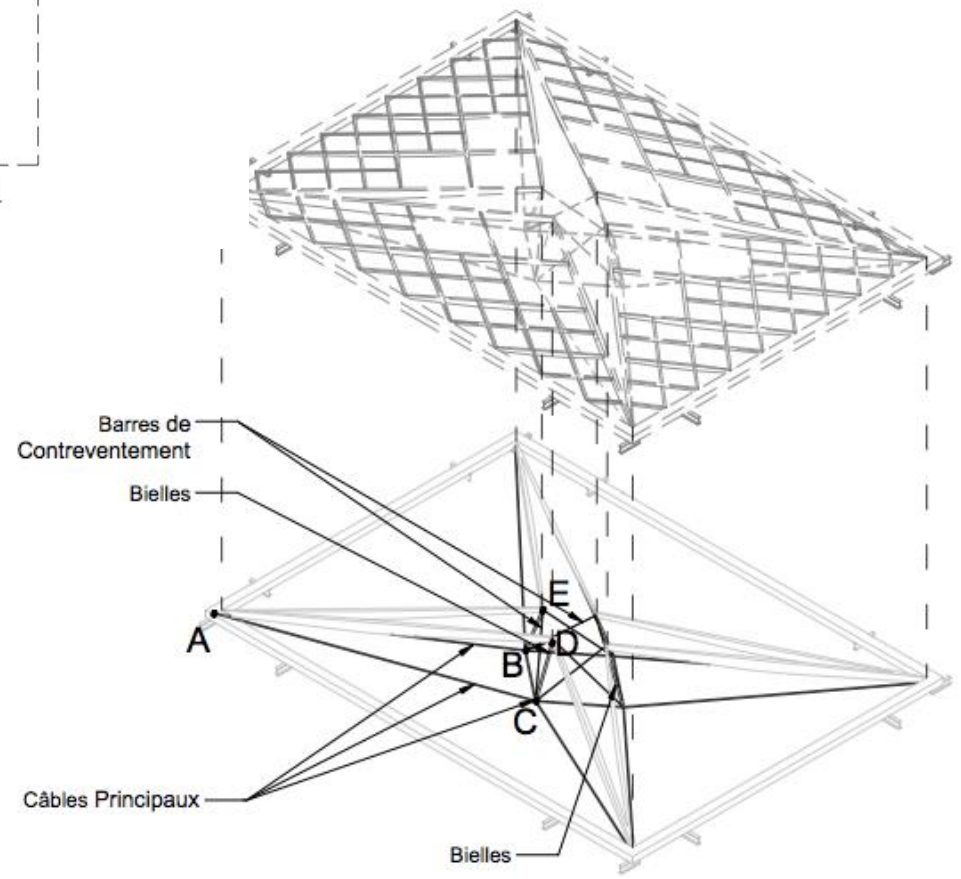
04 VUE PERSPECTIVE GEOMETRIE CABLES
